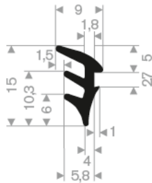
216.03.551 EPDM 65° Shore rollengte 200 meter
