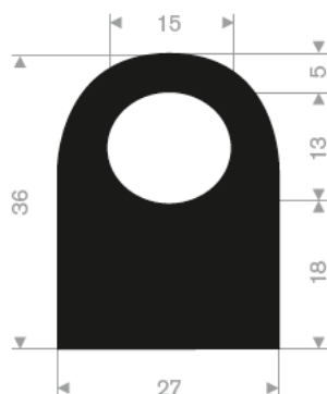
215.28.736 hardheid 40° Shore rollengte 20 meter
